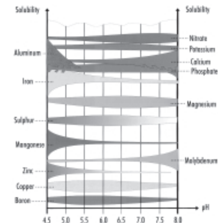
Fig. 2 - Solubilidad de los elementos de acuerdo con valores de pH variables.
