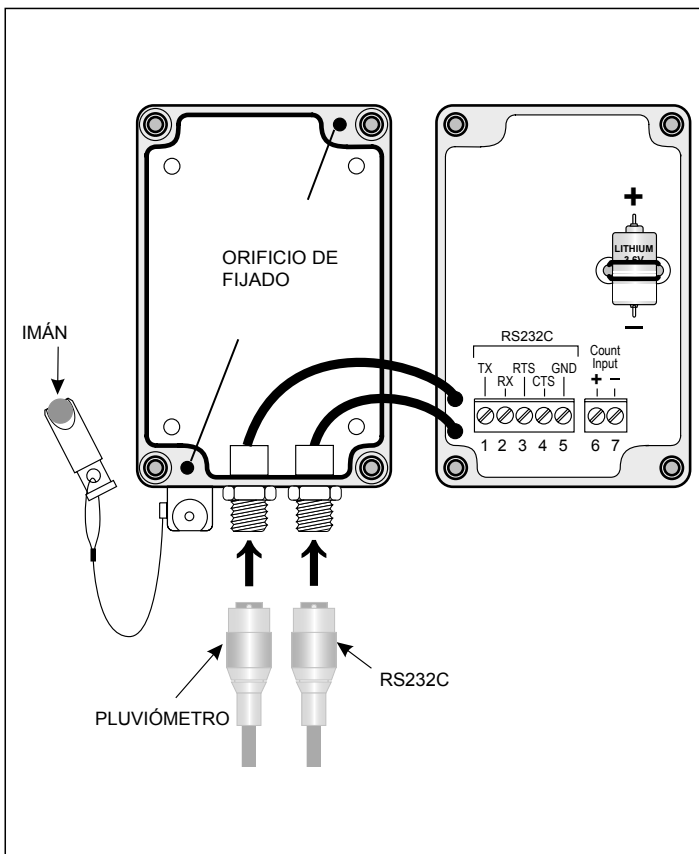
Fig. 6 Interior del instrumento.
